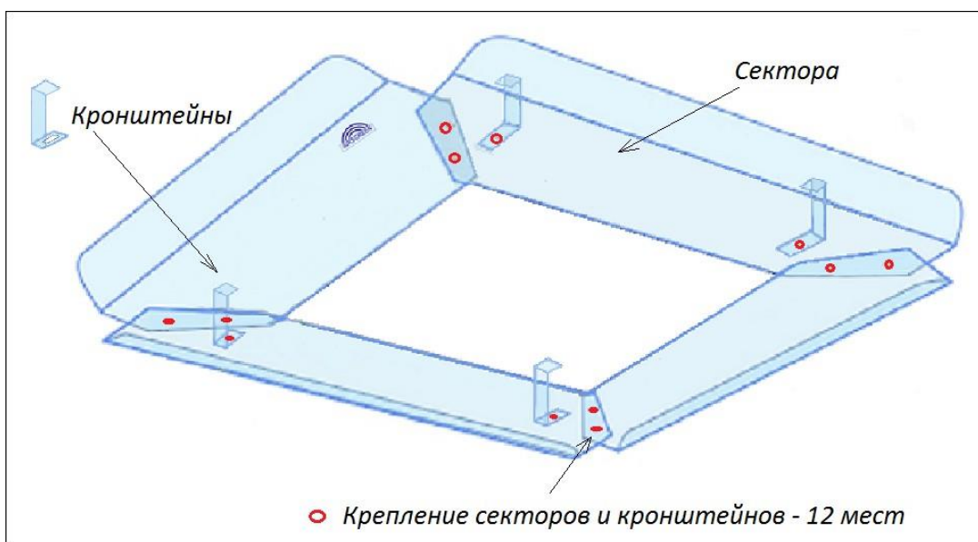
Места крепления. Рис.1
